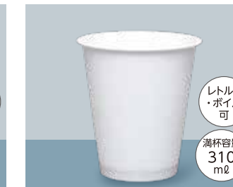
製品名 TS 88-96-310 サイズ 口径:87.5 全高:96.5 (mm) 首下径:80.8 底径:54.7 ケース入数 840 個 加飾 インモールドラベル
